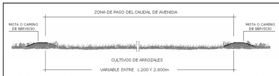
FIGURA 12. Sección tipo del corredor verde de la Marjal Sur.
