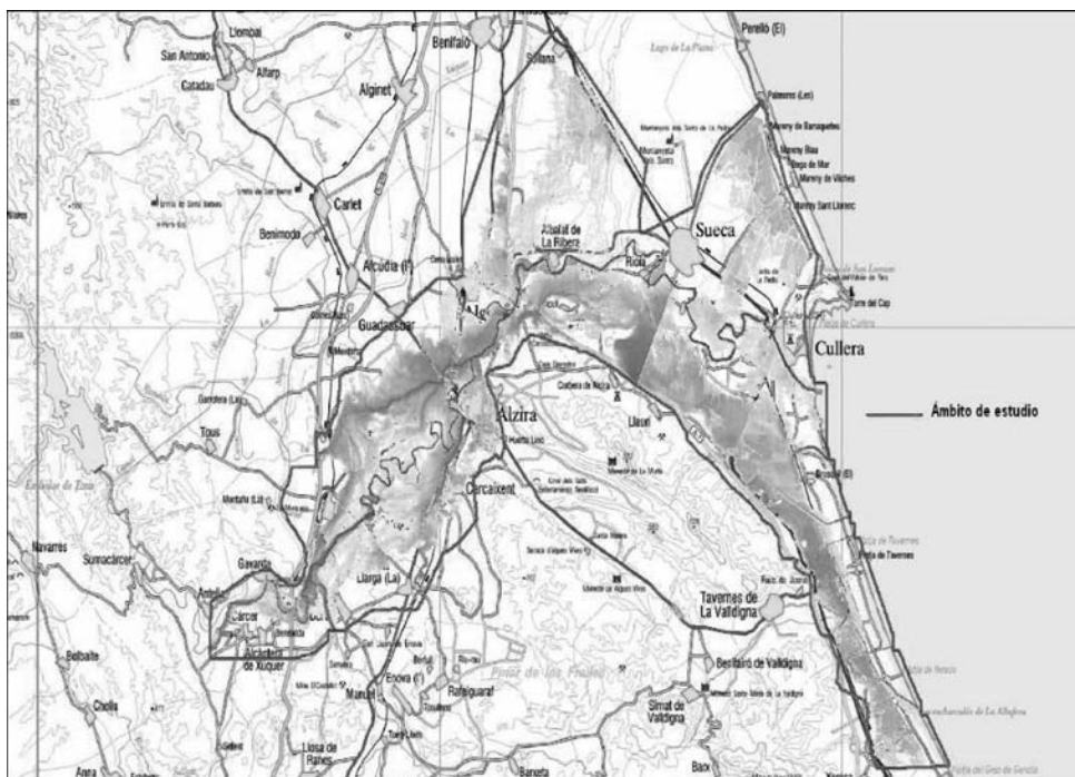
FIGURA 4. Simulación de calados para la avenida de periodo de retorno de 250 años en la alternativa base (situación actual + presas de laminación).
